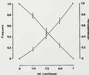
Abb. 3. Normierte Frequenz (O—O) und Periode (▲—▲) an 5 Zeitpunkten der Ruhelaute von Desmodus rotundus murinus ( \bar{x} \pm s )
